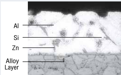
ภาพตัดโครงสร้างทางจุลภาคของเหล็กเคลือบโลหะสังกะสี Microstructure cross section of ZINCALUME® steel
